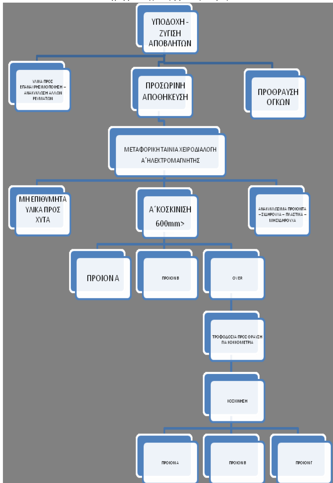
Διάγραμμα Ροής Επεξεργασίας Αποβλήτων
